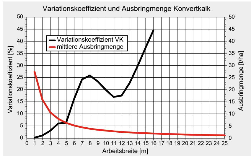
Abbildung 5: Variationskoeffizient und Ausbringungsmenge in Abhängigkeit von der Arbeitsbreite
