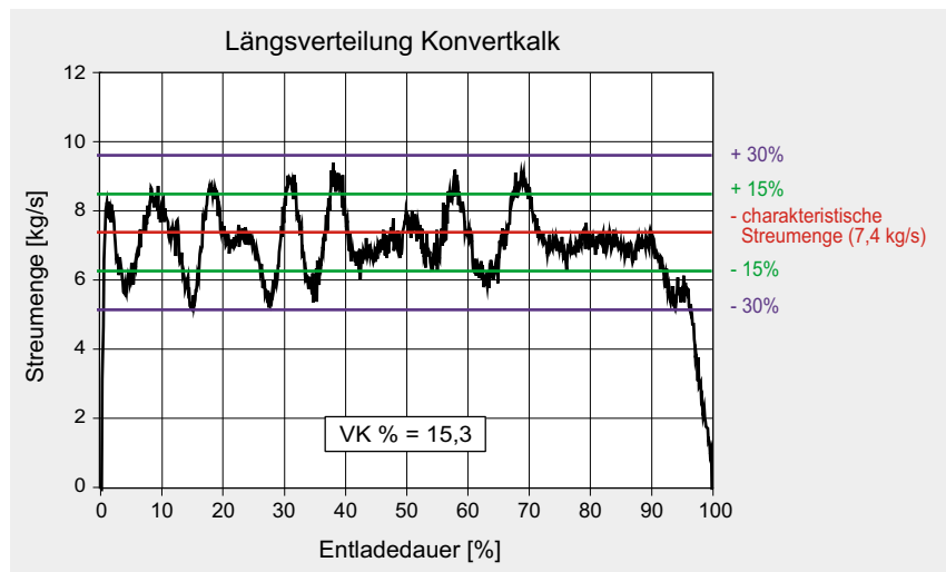
Abbildung 6: Längsverteilung mit Konverterkalk
